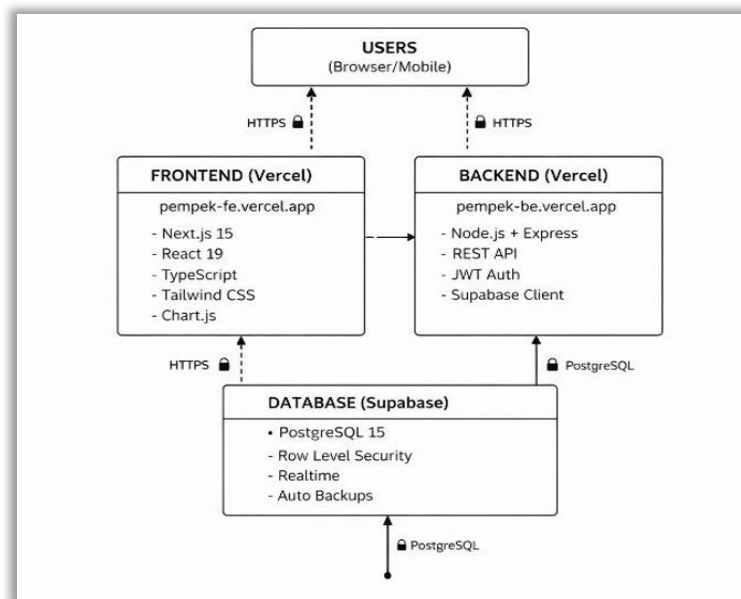
Gambar 4.1 Arsitektur Sistem
